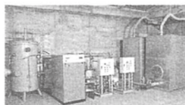
地下水浄化装置
