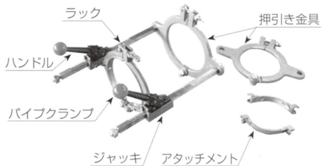
150型（呼び径125・150用）
