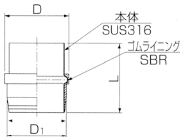
呼び径40・50
