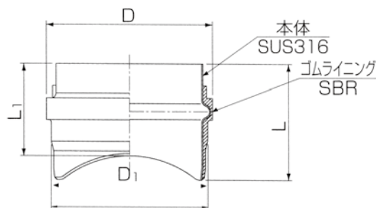
呼び径75・100・150
