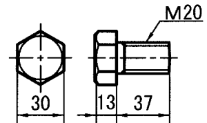
押しボルト (SUS304系)
